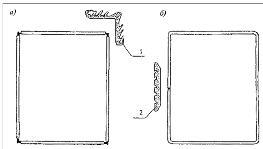
а - дистанционная рамка из прямолинейных деталей, собранная на четырех соединительных уголках (1); б - дистанционная рамка, изготовленная методом гнутья и замкнутая на одном соединителе (2)
