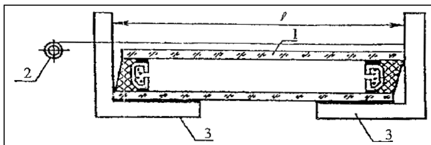
1 - стеклопакет; 2 - рулетка; 3 - угольник; L - контролируемый размер
